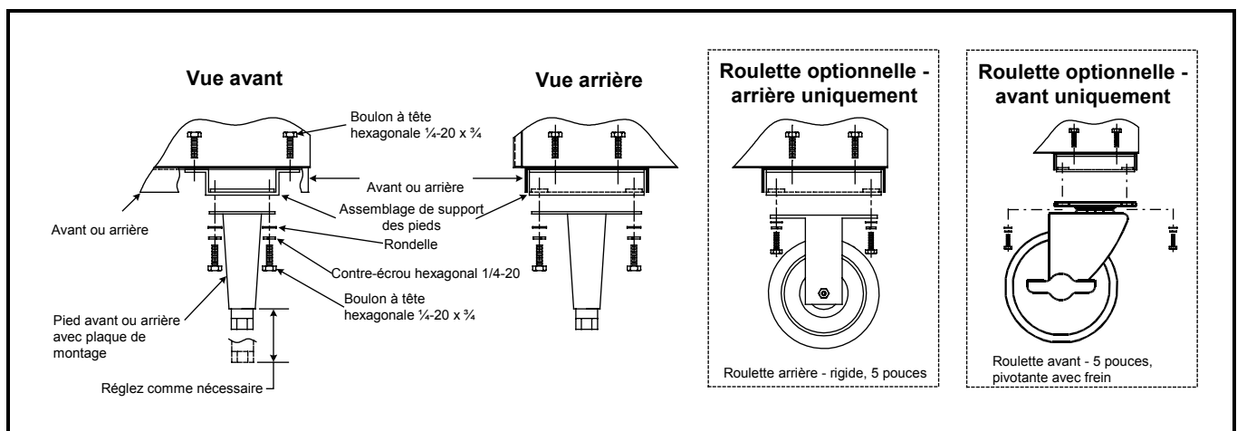
Installation de montage des pieds et roulettes (en option)
