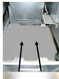
Figure 2 : Positionner le dispositif de fonte dans l'armoire et insérer les languettes dans les fentes du guide d'alignement.
