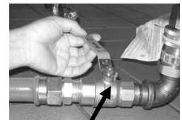
Vanne manuelle
